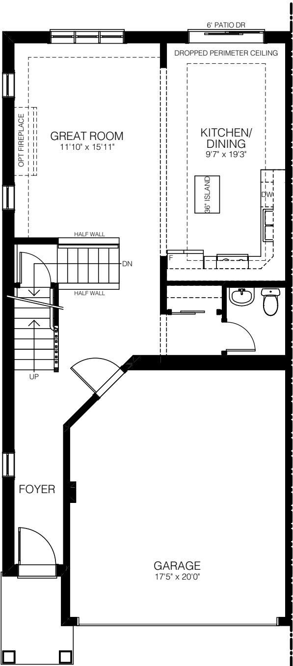
MAIN FLOOR ELEV. M1/M2/M3/M4
